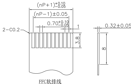
FPC软排线
